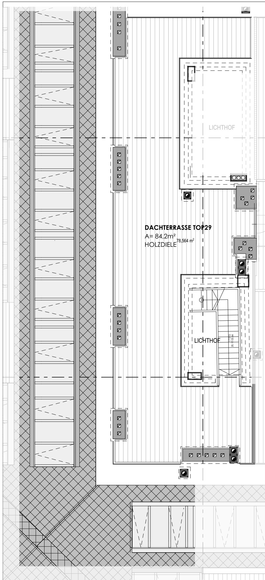
6. Dachdraufsicht 1:500
